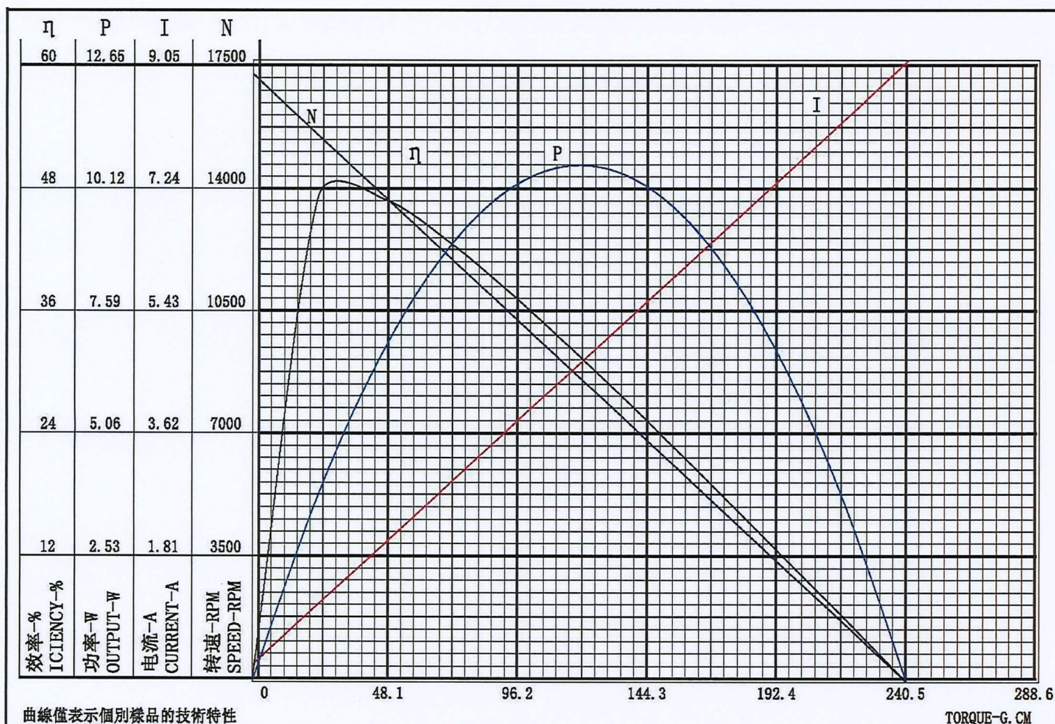
马达全功能测试曲线图
